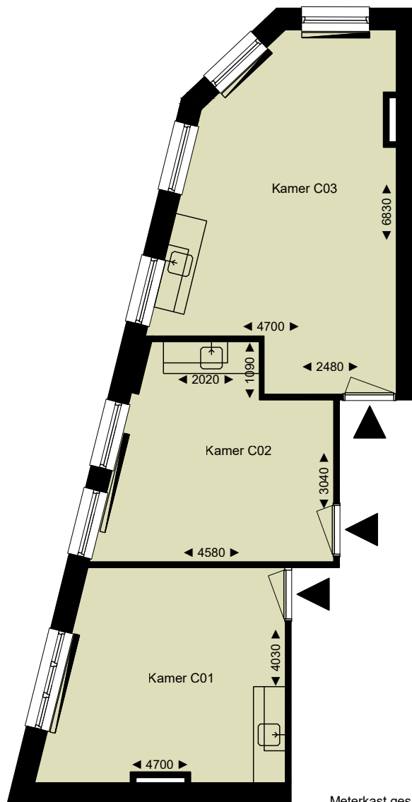
2e verdieping schaal 1:100
