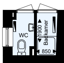
2e verdieping schaal 1:100
